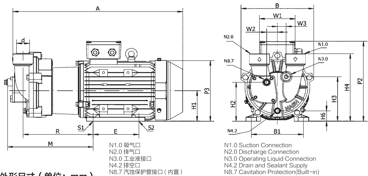
外形尺寸 (单位: mm)
