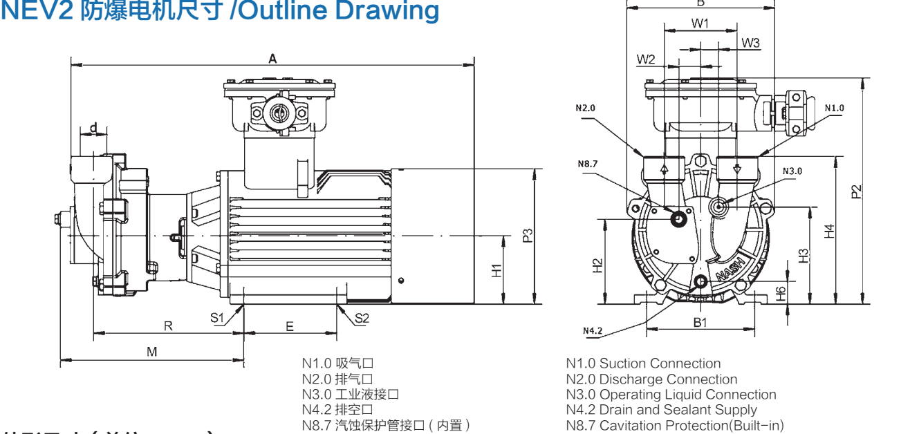
外形尺寸 (单位: mm)
